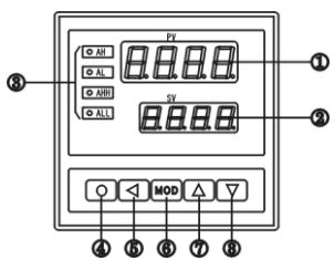
1 面板及按键说明 (以96×96尺寸的仪表为例)
